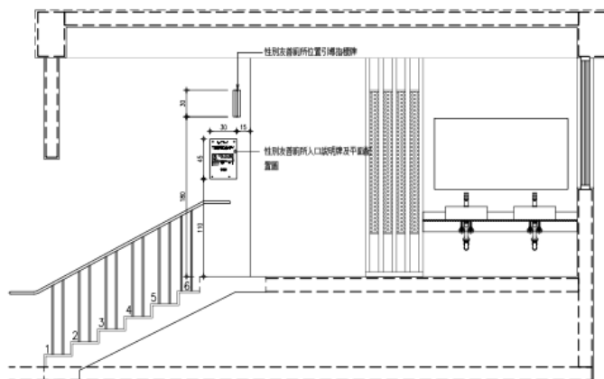
④ A4 活動中心性別友善廁所外牆施工立面圖
