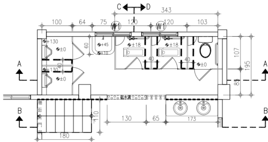
① A4 活動中心性別友善廁所設計平面圖
